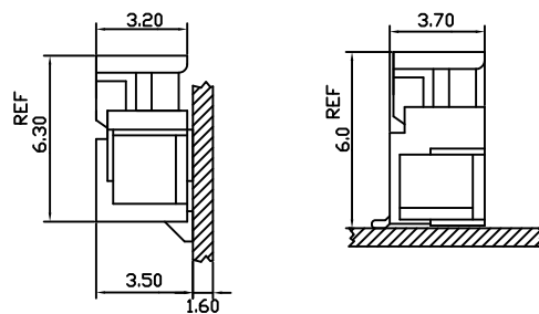
SMT TYPE
