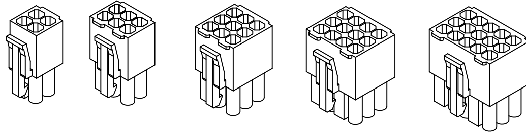
E130H-04(2X2) E130H-06(2X3) E130H-09(3X3) E130H-12(3X4) E130-15(3X5)
