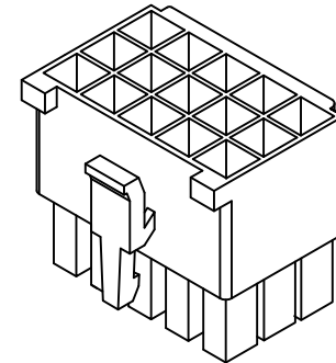
E158H-15A (3X5)
