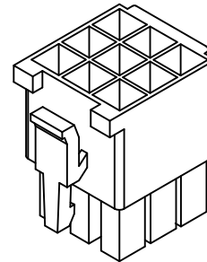
E158H-09A (3X3)
