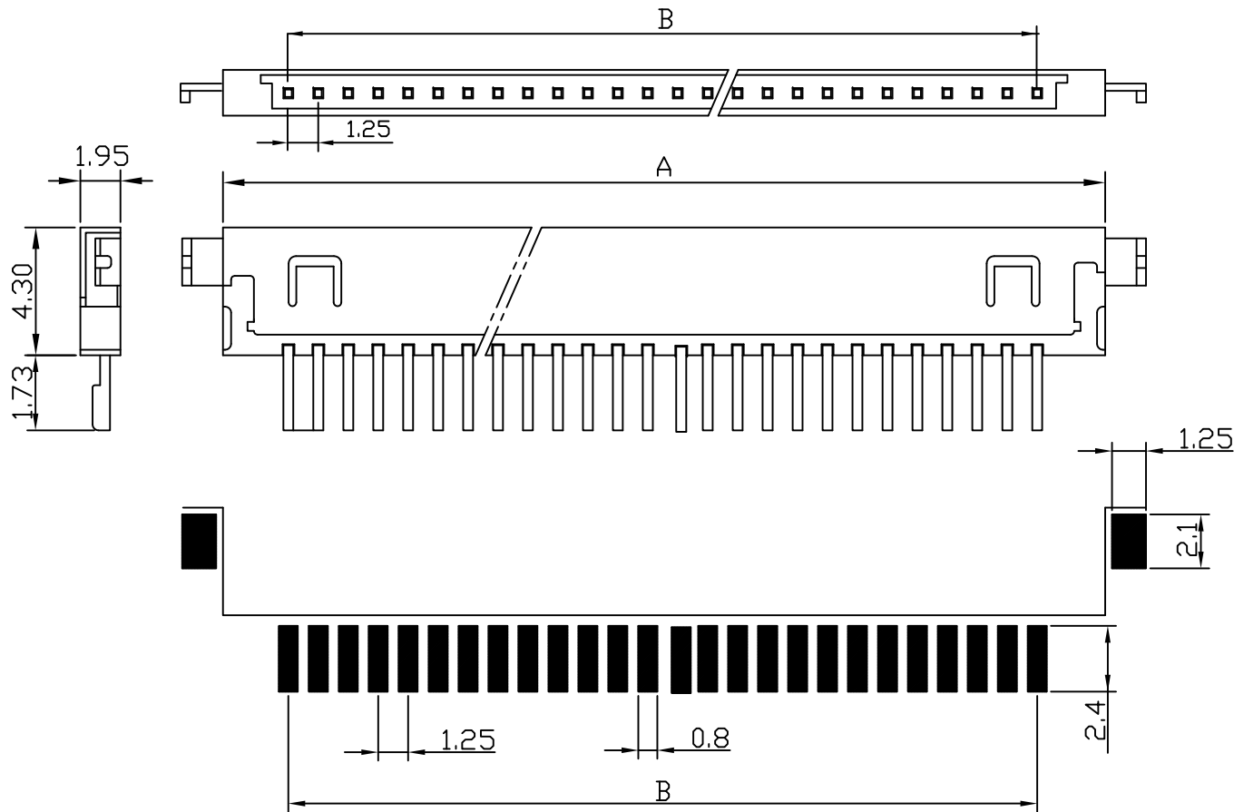
P.C LAYOUT
